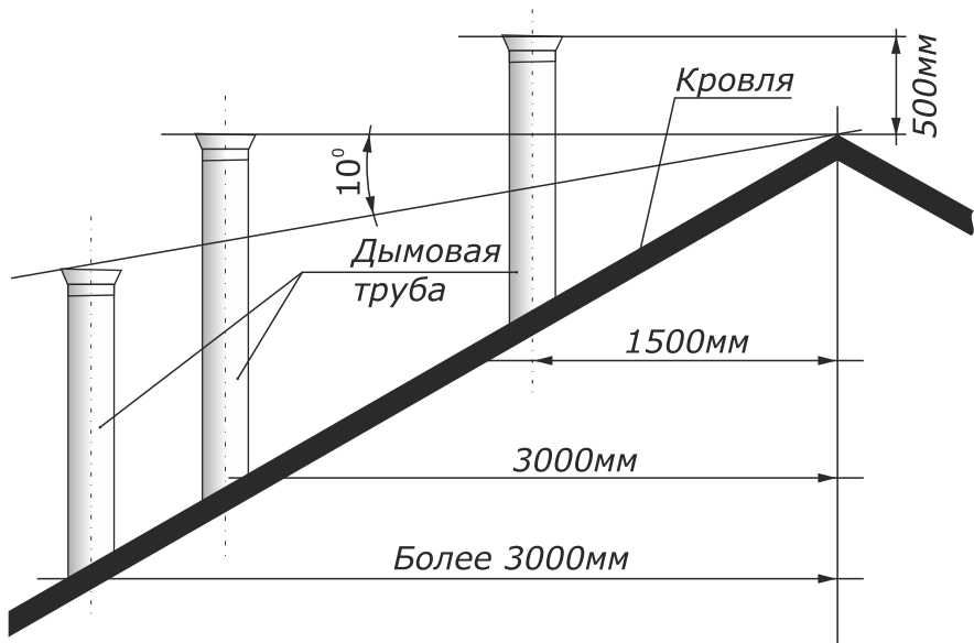
Рис 1. Возвышение дымовых труб над кровлей
